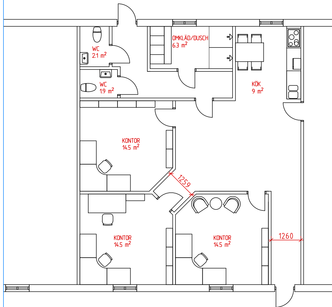
FÖRSTORAD PLANVY ÖVER MITTEN SKALA 1:50
